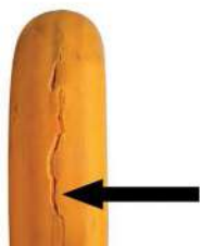
° La rueda de la competencia falló con un fuerte agrietamiento de la banda de rodadura después de solo 4.7 millas.
